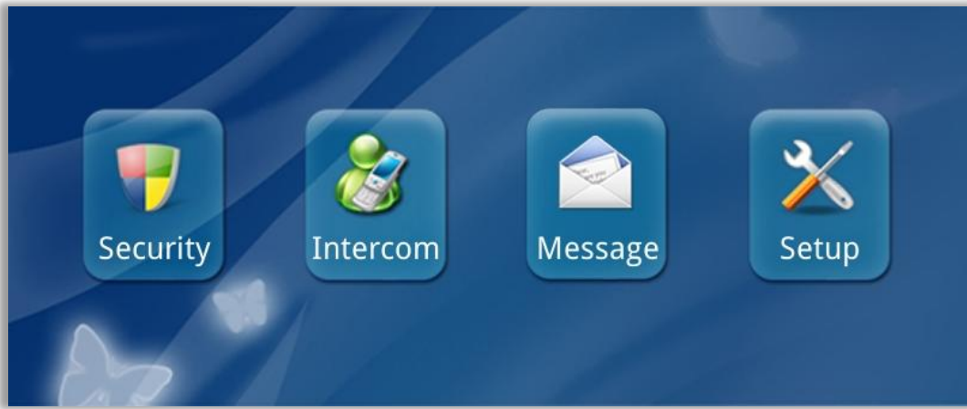
Fig. 11 : Menu Bar
