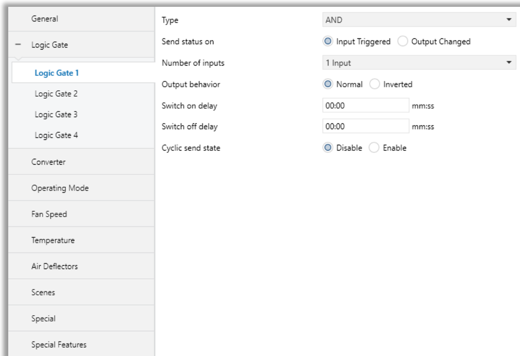
Fig. 8: Logic Gate X Configuration Parameter Page
