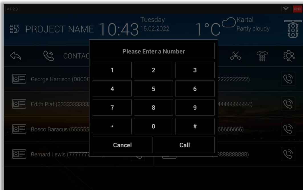
Fig. 45: Dialer Window
