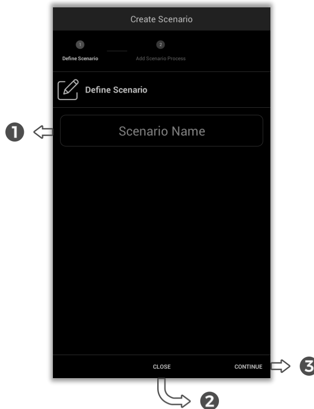
Fig. 33: Create Scenario - Define Scenario
