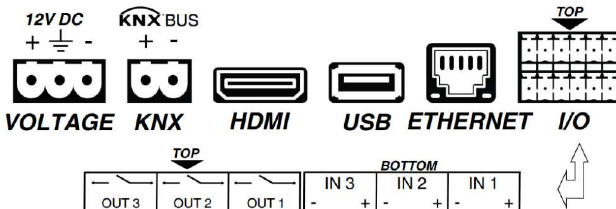
Fig. 3 : Connectors
