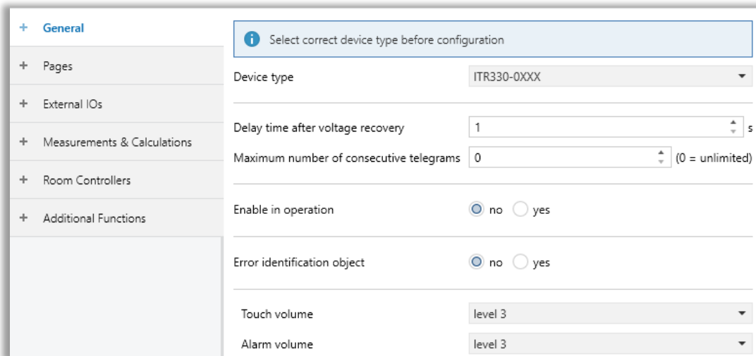
Fig. 4: General Parameter Configuration Page
