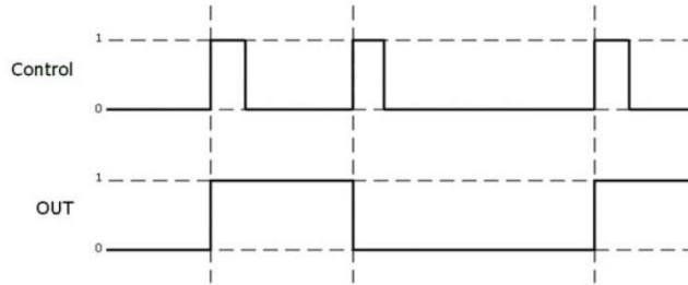
Fig 14 : Rising Edge Behaviour
