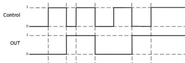
Fig 13 : Falling Edge Behaviour
